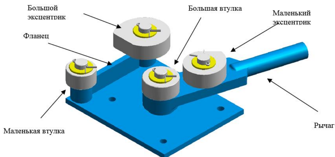
Деталировка гибочной машины DR-25
