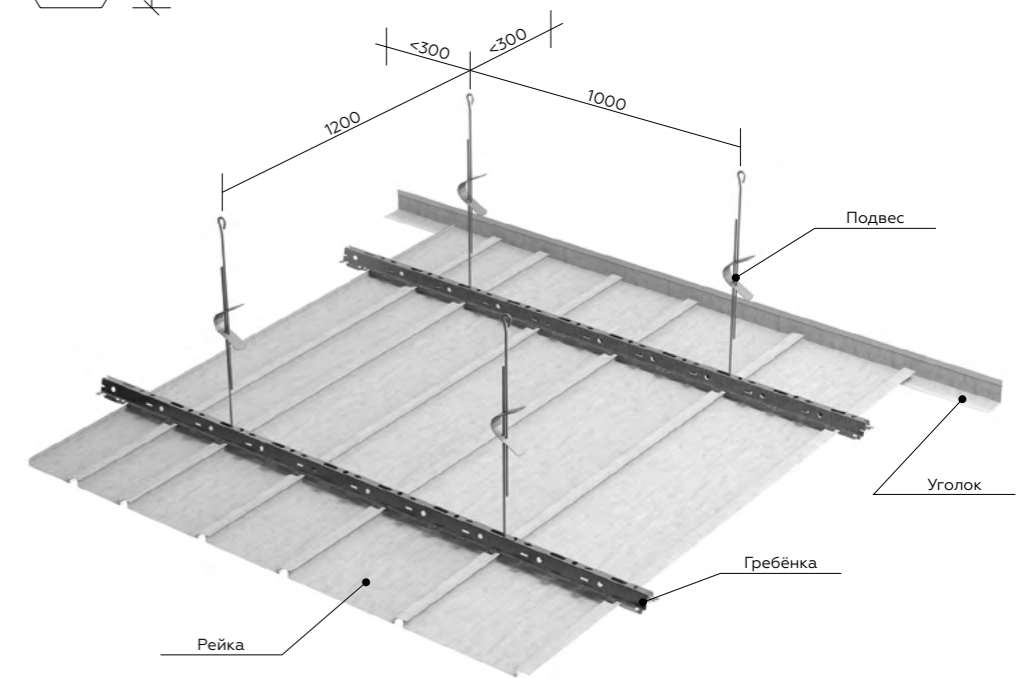
Закрытый стык реек
