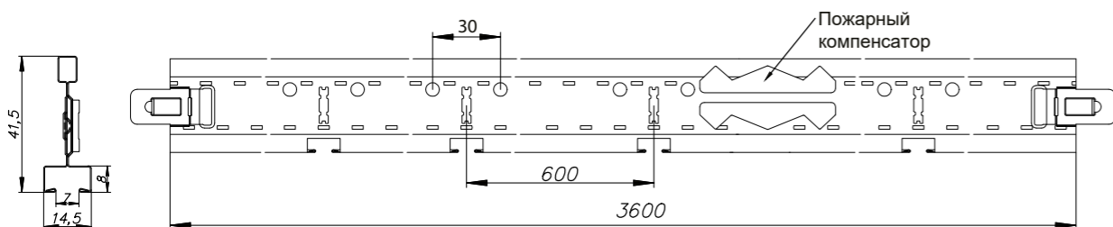
Профиль несущий основной 14,5/41,5 L=3600
