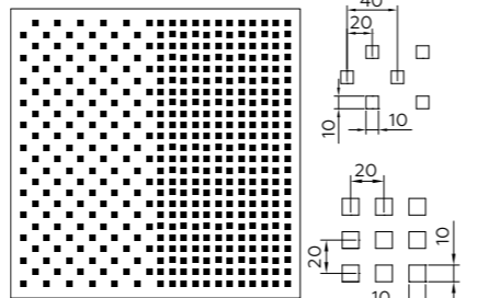
K45 | K90 % перф. 12,5 | 25 мини-квадраты (10x10 мм)
