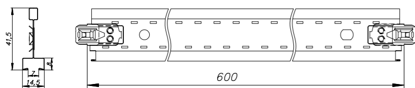
Профиль несущий вспомогательный 14,5/41,5*** L=1200
