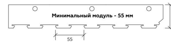
Гребёнка ВТ 19
