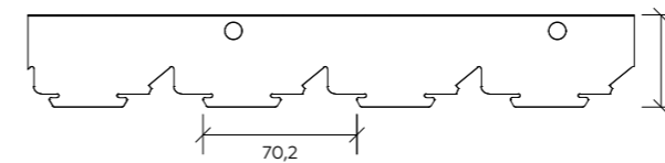
Гребёнка ВТ 4-70
