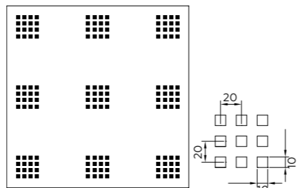
K9 девять квадратов (60x60 мм)
