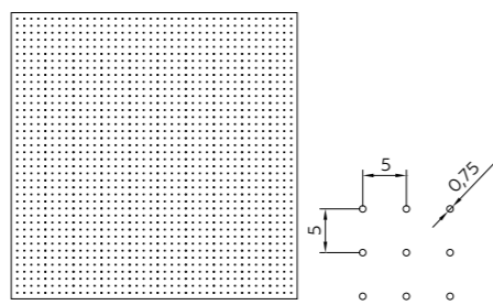
F90 (d=0,75/5 мм) % перф. 2
