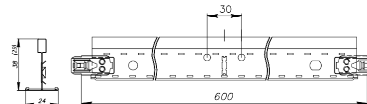
Профиль несущий вспомогательный 24/29, 24/38** L=1200
