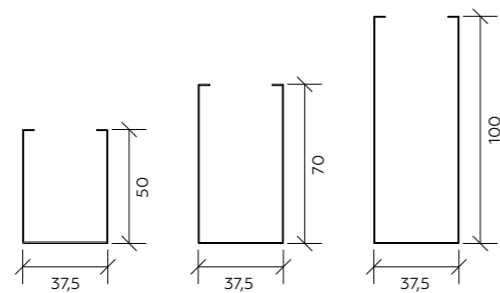
Гребёнка ВТ 4-70
