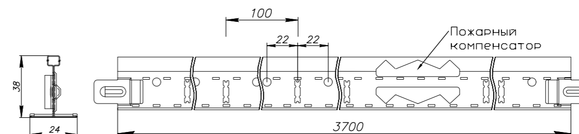
Профиль несущий основной 24/38 L=3700
