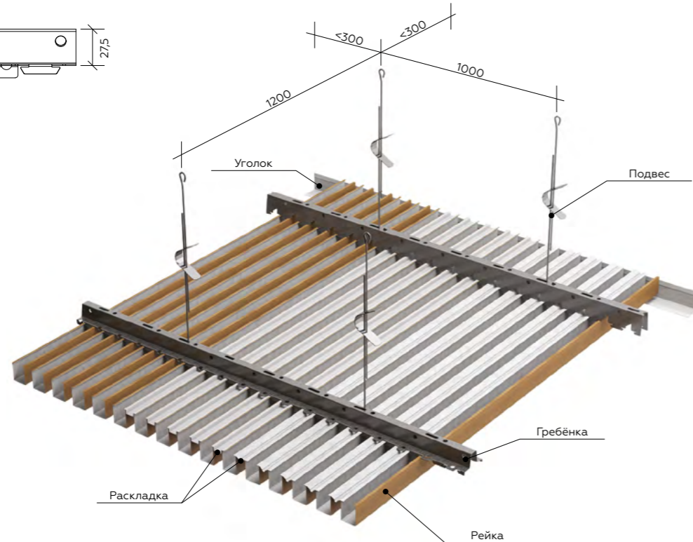
Гребёнка ВТ 12-50
