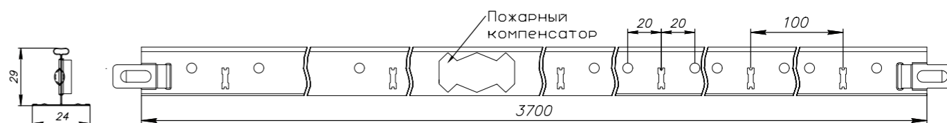
Профиль несущий основной 24/29 L=3700
