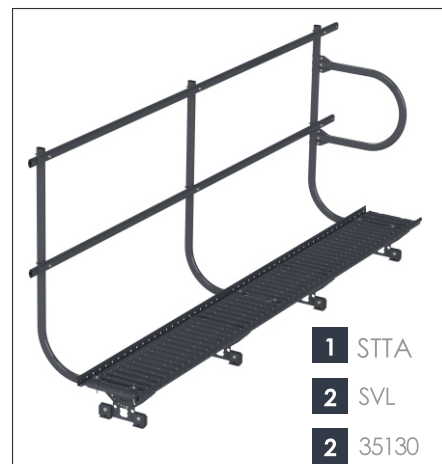
ПЕРИЛА К КРОВЕЛЬНОМУ МОСТИКУ SVL 3 м (H=1,1 м)
